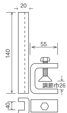
水平金具
