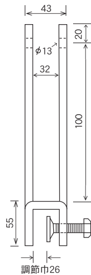
垂直金具
