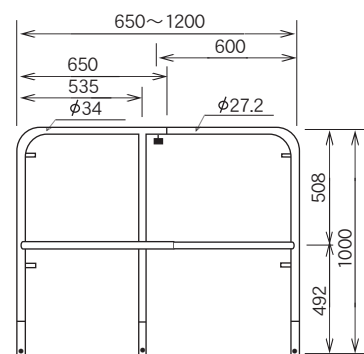
ST4型
