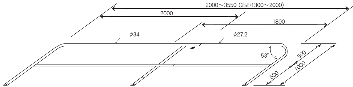
ST1・2型
