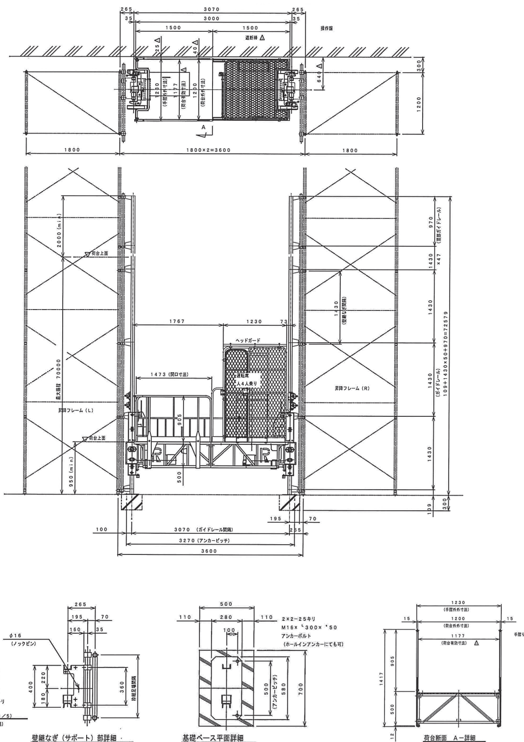
主要寸法図 (単位: m/m)
