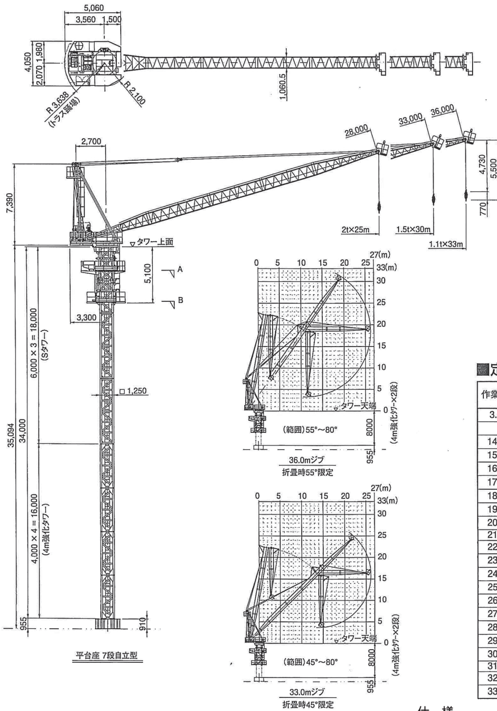
主要寸法図 (単位:m/m)
